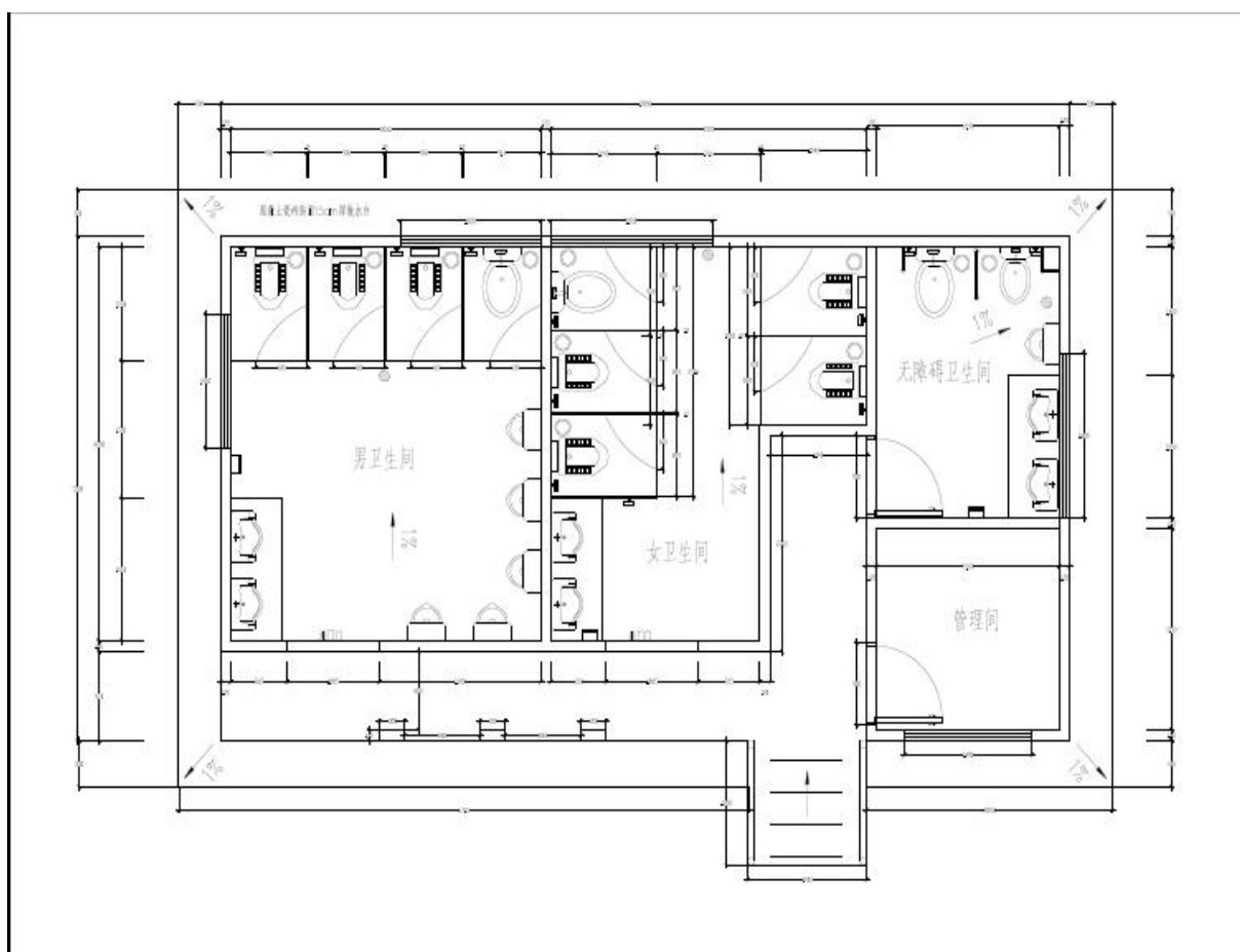
博鳌火车站旅游厕所平面图
