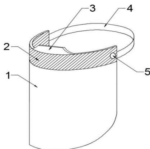
1、弧形面罩、2、标贴、3、泡沫条、4、松紧带、5、树脂扣
