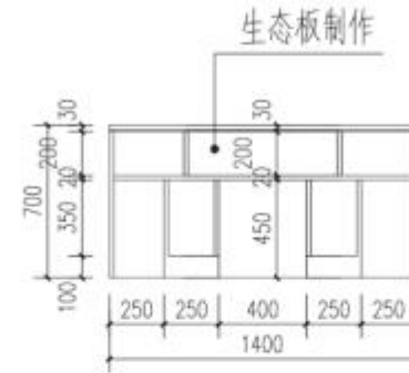
六边桌立面图 1:50
