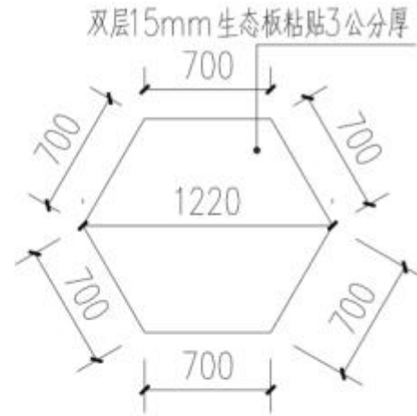
③九 六边桌 1:50
